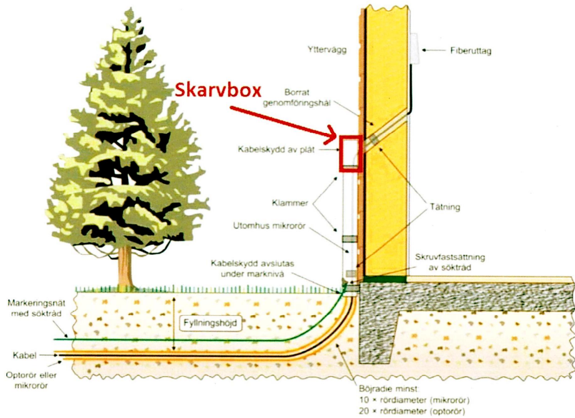
Figur 2. Utförande av fiberinstallation.
